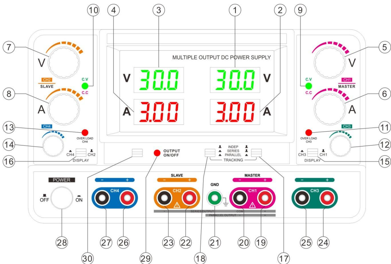
圖 3-1 前面板圖
