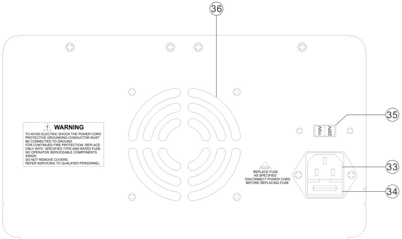
圖 3-2 後面板
