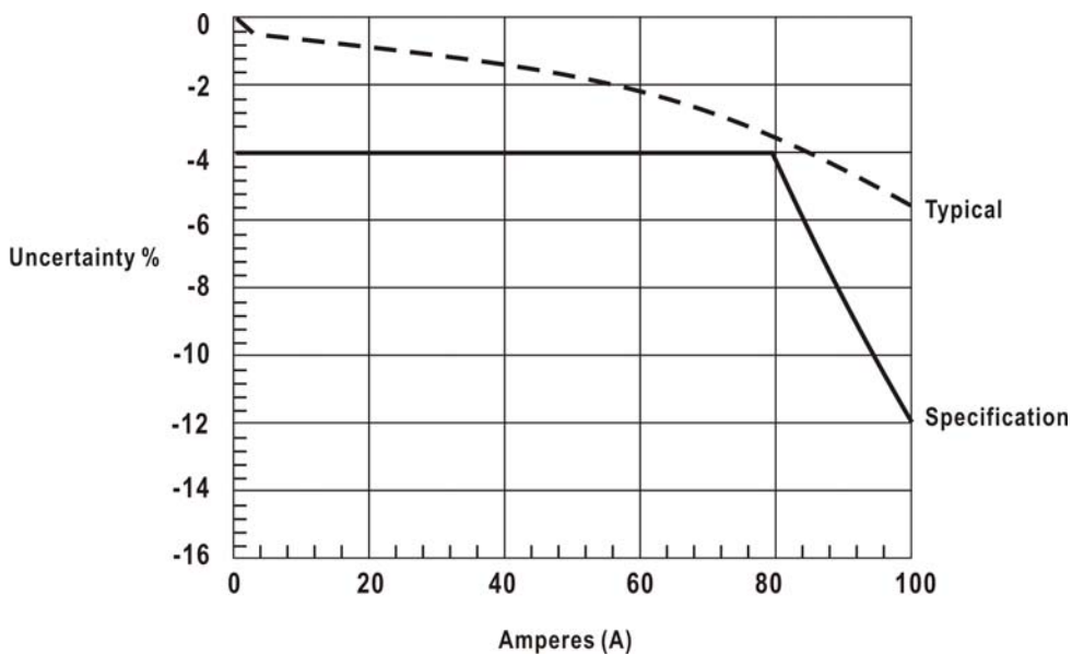
圖 8: 典型的 DC 信號線性在 0.1V/A 範圍時
