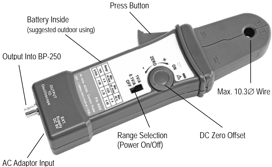
圖 1: PA-699 電流探測鉗上的控制及指示。
