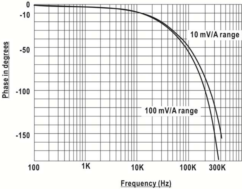
圖 9: 典型的位相對頻率在 1A 峰值時
