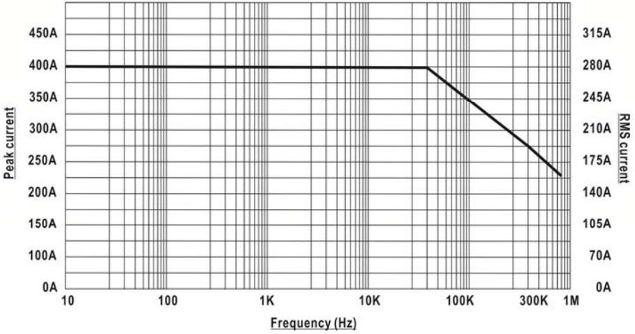
圖 7: 最高電流量對頻率
