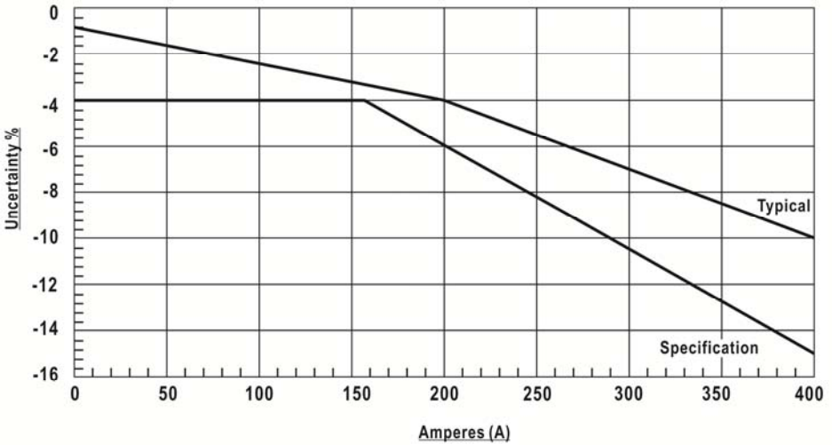
圖 8: 典型的 DC 信號線性在 10 mV/A 範圍時
